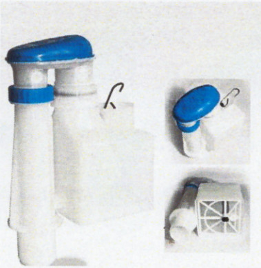
TOILET SYPHON
